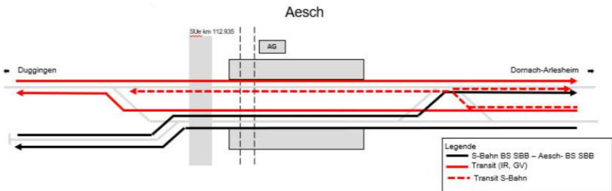
Abbildung 5: Betriebskonzept Aesch Bestvariante [1]
