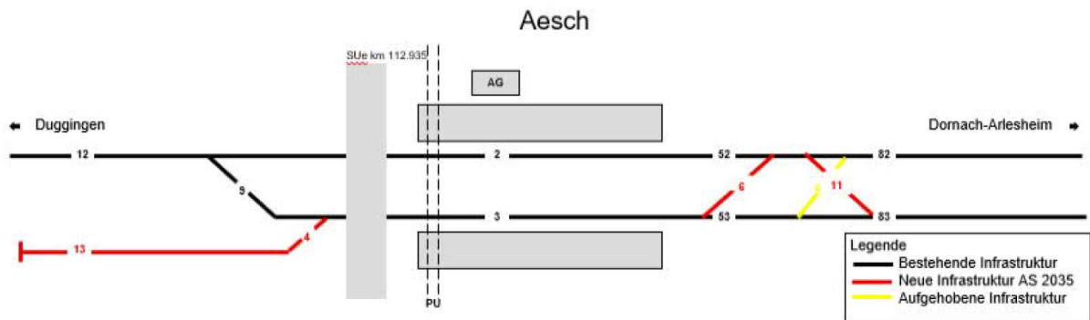
Abbildung 4: Topologieskizze Aesch Bestvariante [1]
